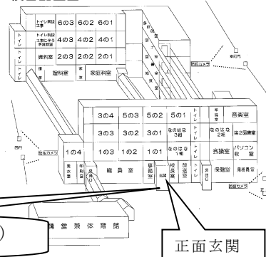
校舎配置図
